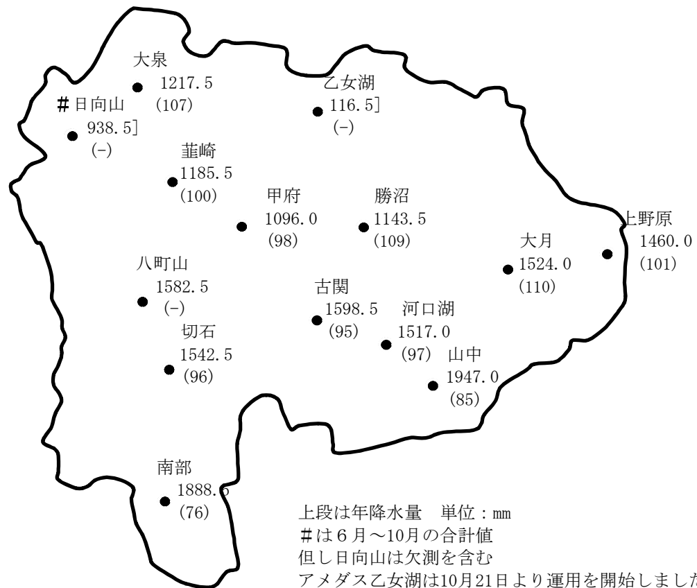
年降水量分布図
