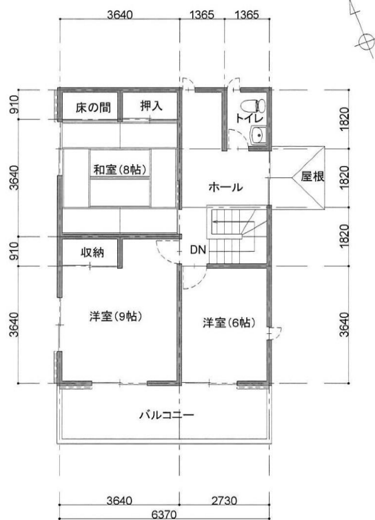
2階平面図
