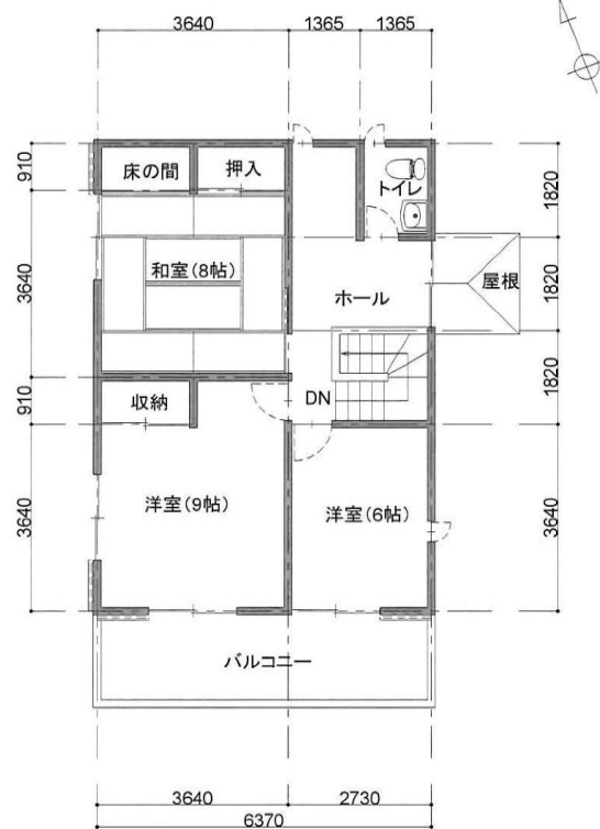
2階平面図
