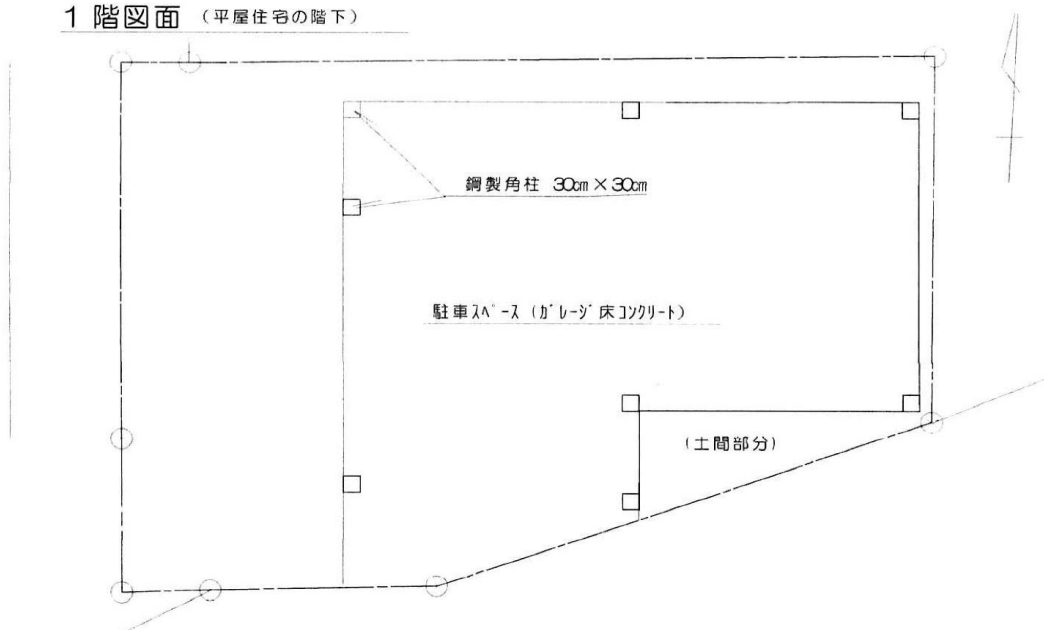
1階図面 (平屋住宅の階下)
