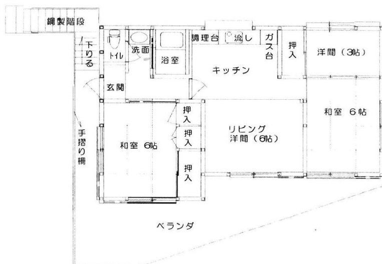
住宅図面 (平屋建)
