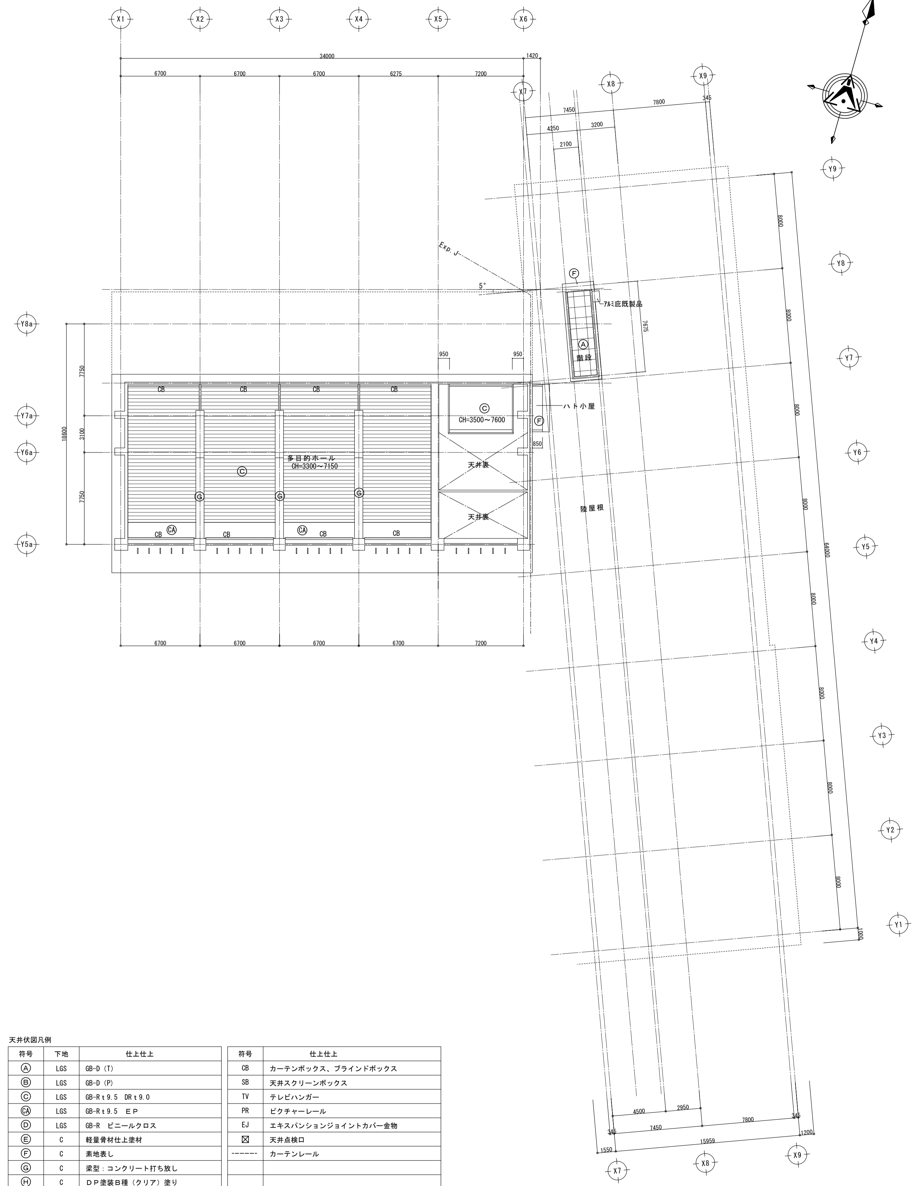
R階天井伏図 S=1:200
